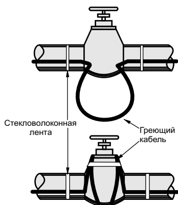
Рис.5 Вентиль. Типичный метод установки
